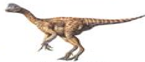
Oviraptor philoceratops
