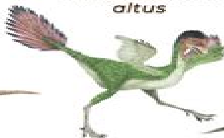
Caudipteryx zoui
