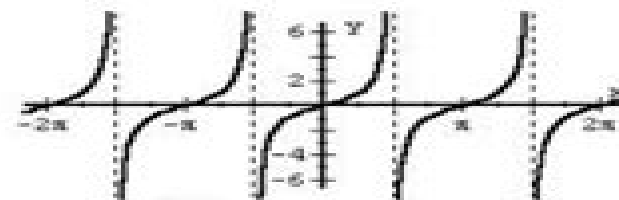
f(x) = \tan x
