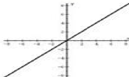
f(x) = x Linear
