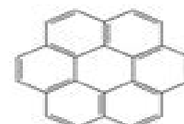
Coronene
