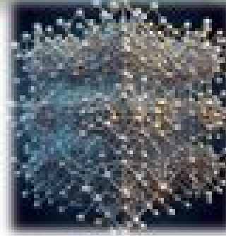
MOF-5
