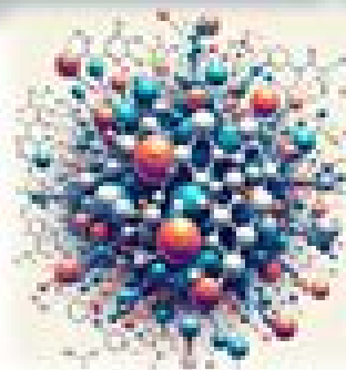
\text{LaNi}_5\text{H}_9
