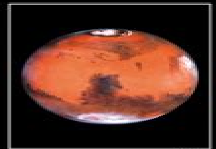
Mars
