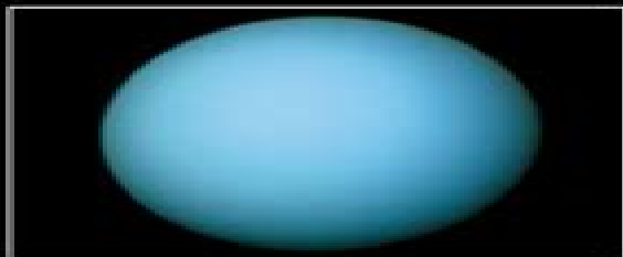
Uranus
