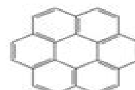
Coronene
