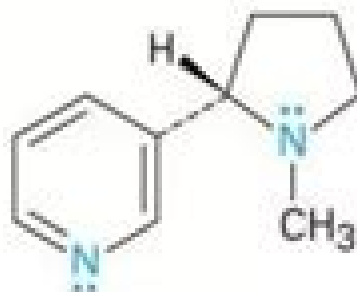
Nicotine
