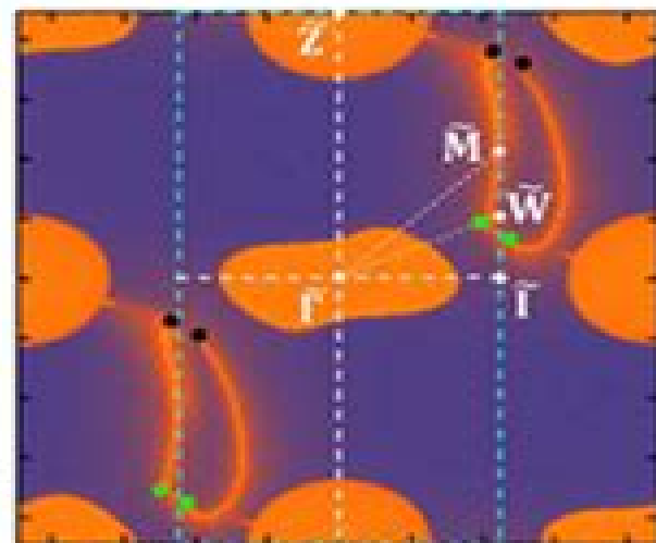
Twin Weyl fermionic pairs
