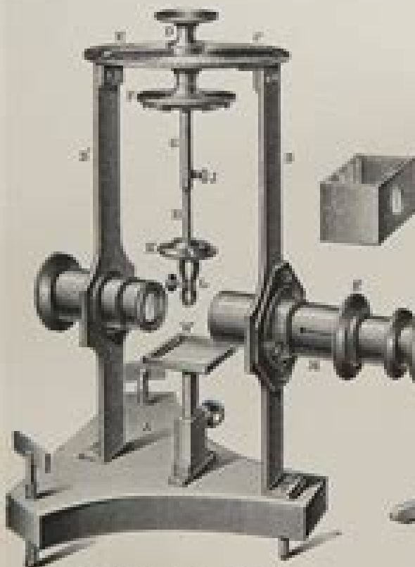
Fig. 11. Achromatisirungsapparat von Lang.
