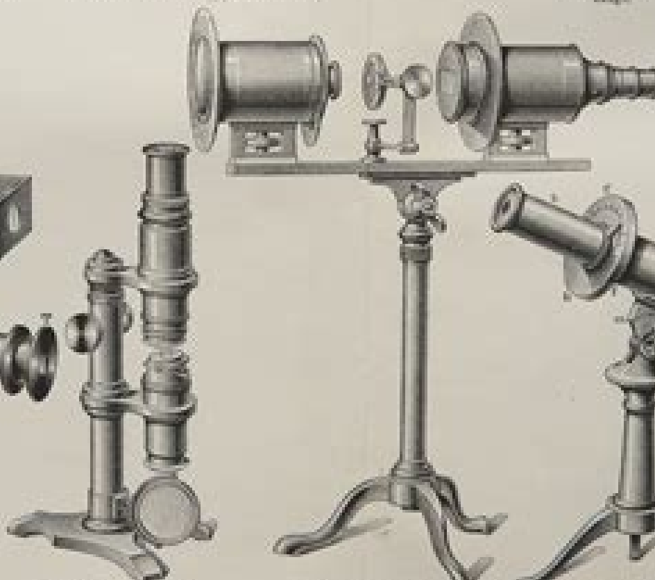
Fig. 12. Mikroskopischer Polarizationsapparat von Helmholtz.
