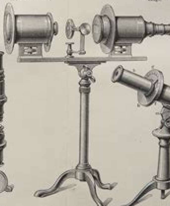
Fig. 13. Objectiv-Polarisationsapparat von Duboy.
