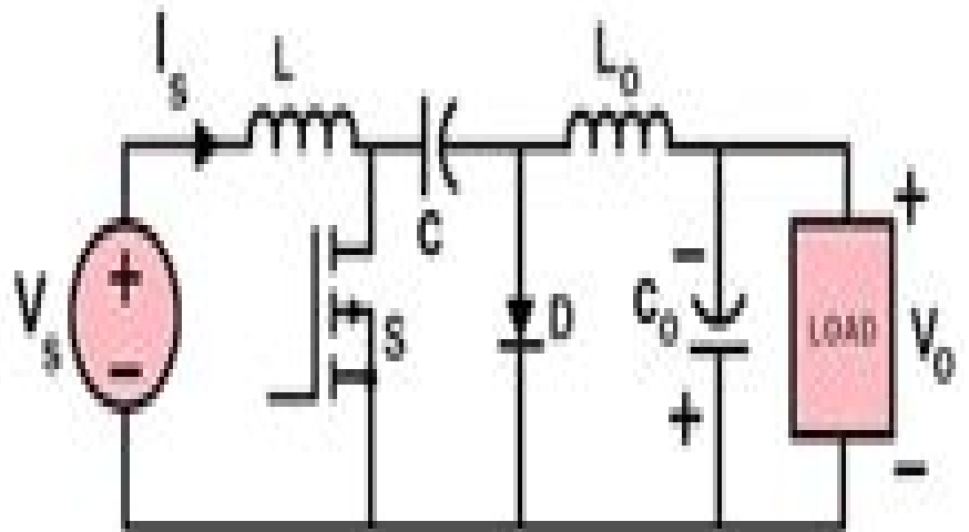
Cuk Converter
