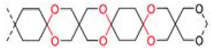
polycycloacetal
