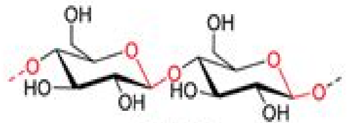
cellulose
