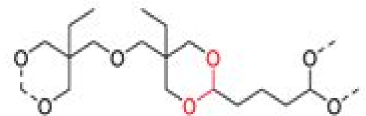
polycycloacetal
