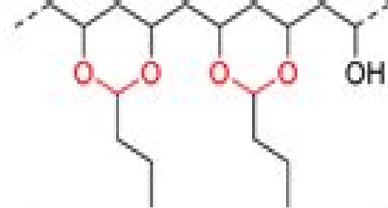
polyvinyl butyral
