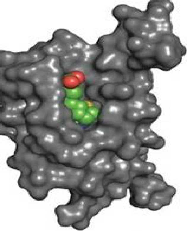
Biotin:avidin
