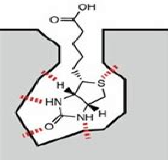
Biotin:avidin
