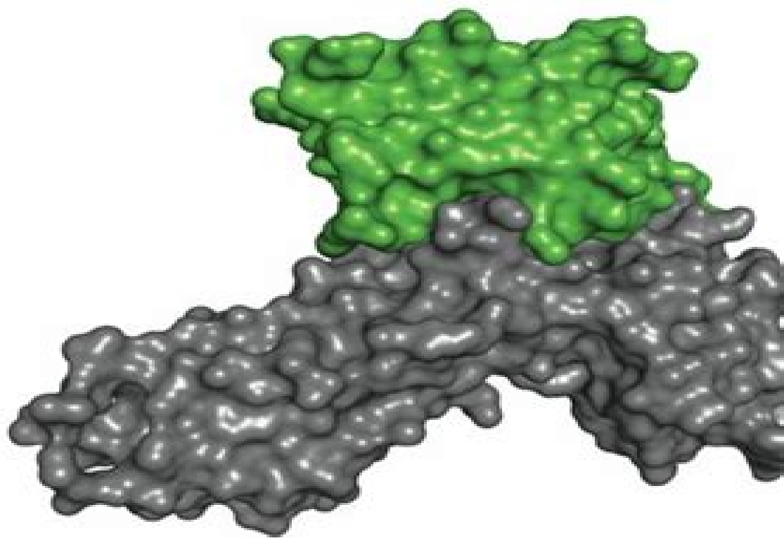
hGH:hGHR
